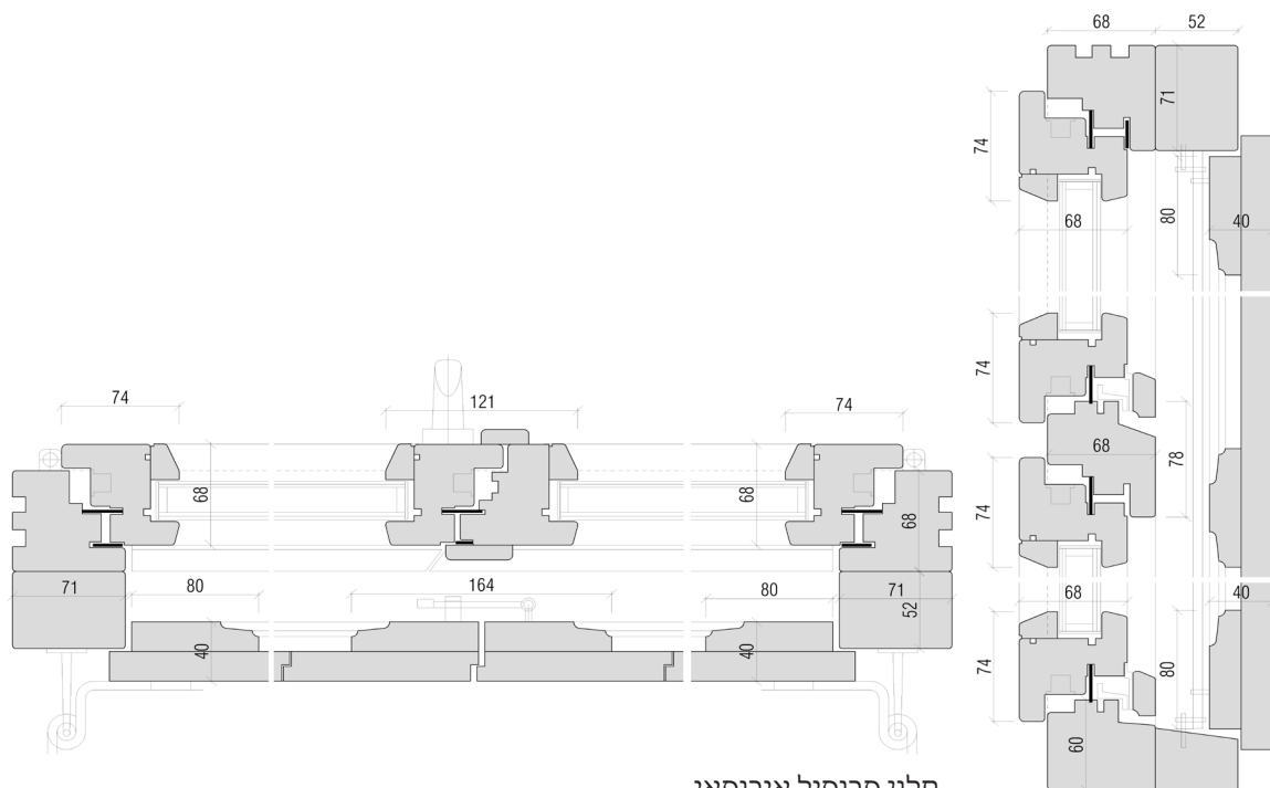
חלון פרופיל אירופאי
